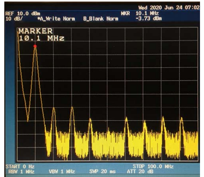
10MHz 70mW送信時 (0~100MHz)
