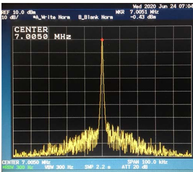
7MHz 100mW時 ( f_0 \pm 50\text{kHz} )
