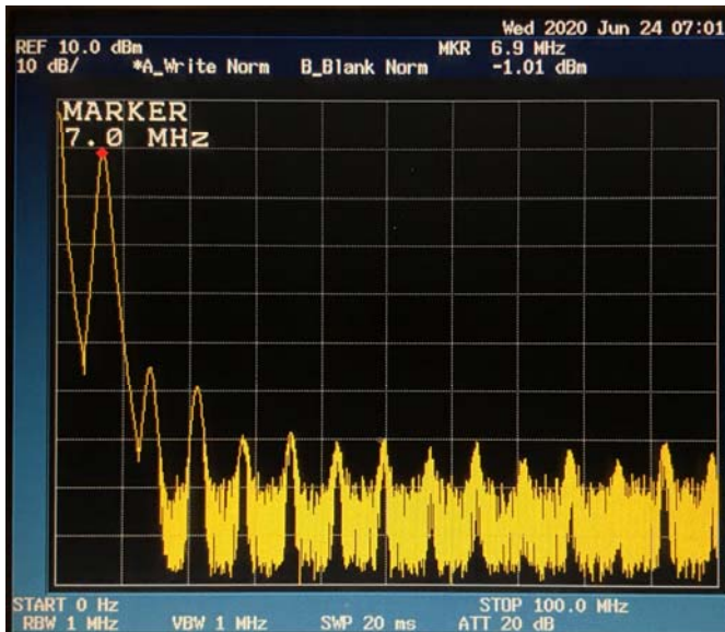
7MHz 100mW時 (0~100MHz)
