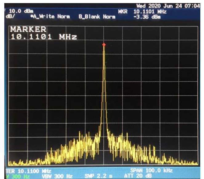
10MHz 70mW送信時 ( f_0 \pm 50\text{kHz} )
